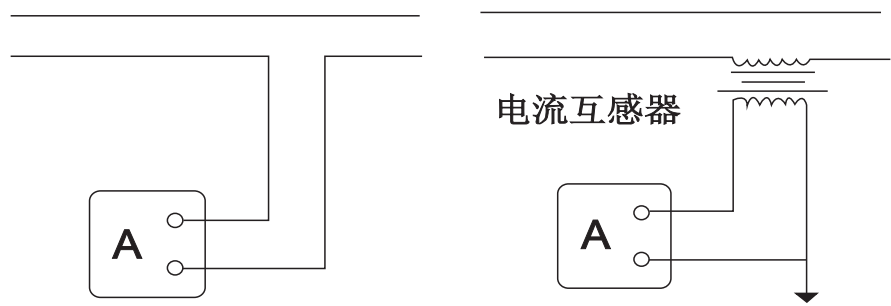
图1 直接接通电流表 图2 经电流互感器接通电流表
