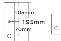
大孔 \Phi 18\text{mm} 、小孔 \Phi 10\text{mm} 底座安装尺寸
