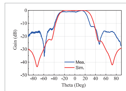
f=15.5GHz 时天线 H 面增益仿真和实测结果对比
