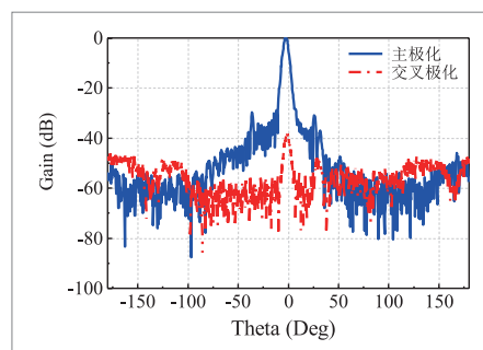
f=15.5GHz 时天线 E 面主极化和交叉极化实测结果对比
