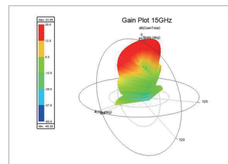
15GHz 波导缝隙阵 3D 方向图
