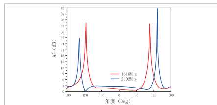
两天线轴比宽度
