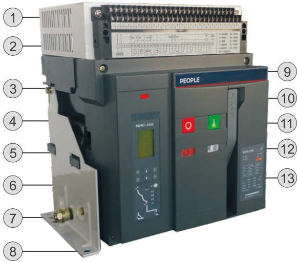
固定式断路器
