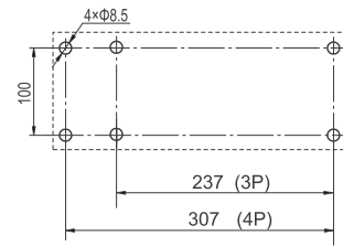
安装尺寸示意图
