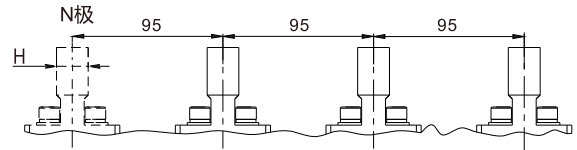
垂直接线及相间距
