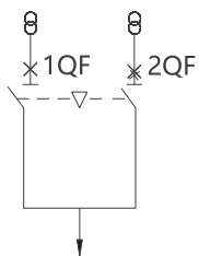
两路电源一路负载只能合一台断路器 电路图
