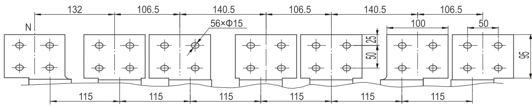
4P水平接线及相间距
