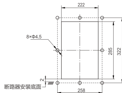
RDW5-1600H固定式断路器面板开孔尺寸
