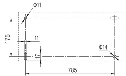
安装尺寸示意图
