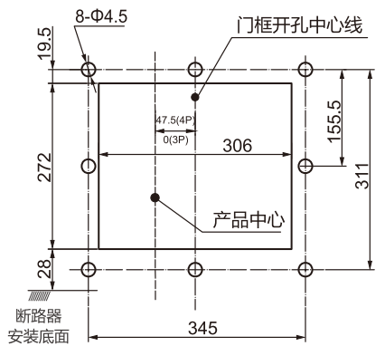
RDW5-2000H固定式断路器面板开孔尺寸
