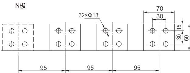
水平接线及相间距
