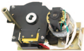
RDW5-2500~6300(S)储能电机
