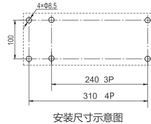
安装尺寸示意图
