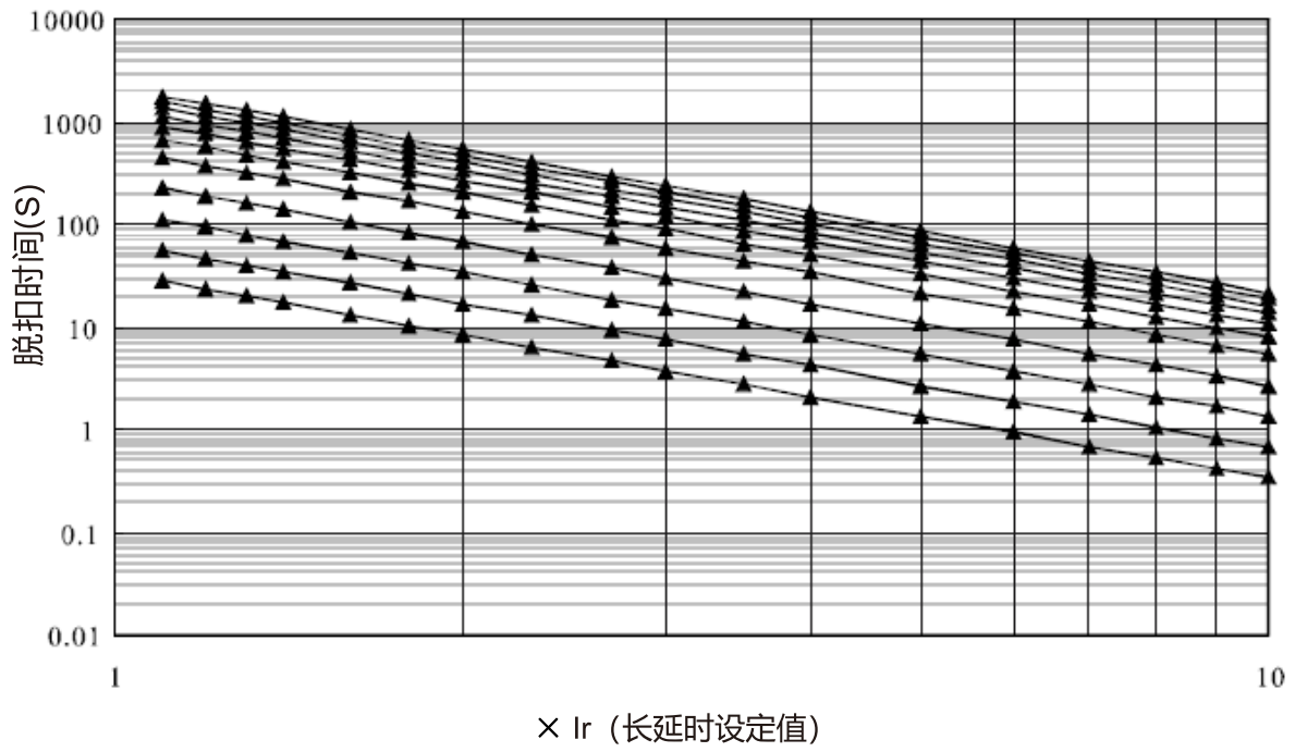
I 2 T 曲线图
