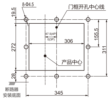
RDW5-2500S固定式断路器面板开孔尺寸
