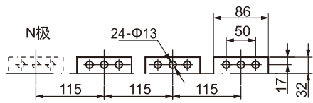
水平接线
