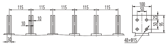
3P垂直接线及相间距
