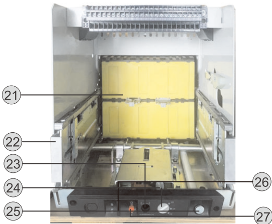
抽屉座
