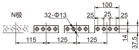
水平接线
