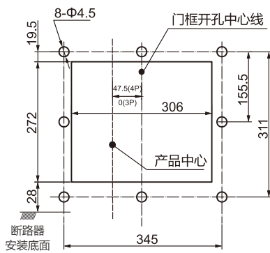
RDW5-2500H固定式断路器面板开孔尺寸
