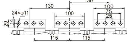
2900-3200 (3P) 水平接线
