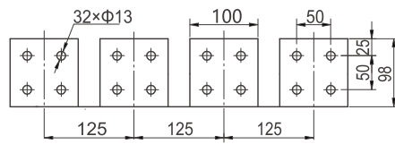
水平接线及相间距
