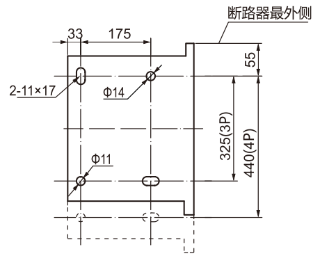
安装尺寸示意图
