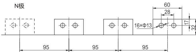
水平接线及相间距
