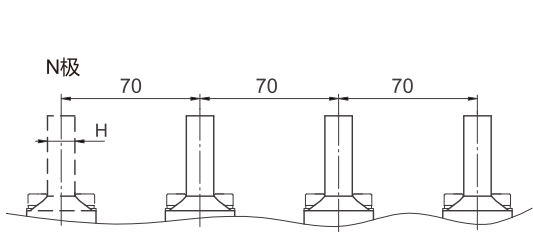
垂直接线及相间距
