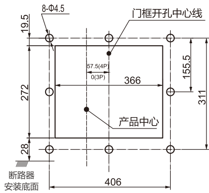
RDW5-3200S固定式断路器面板开孔尺寸
