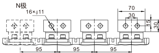
水平接线及相间距
