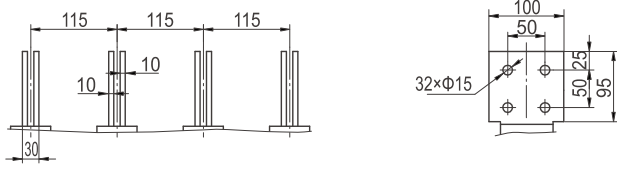
垂直接线及相间距
