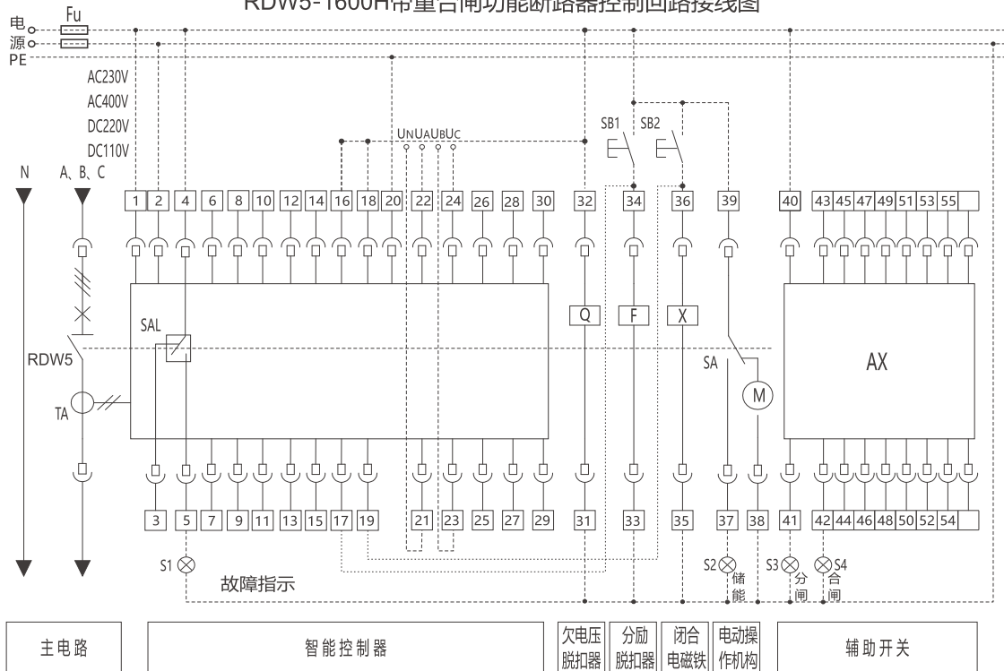
RDW5-1600H带重合闸功能断路器控制回路接线图
