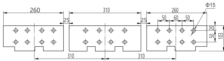
三极水平接线及相间距
