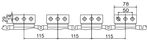
2000-2500 (4P) 水平接线
