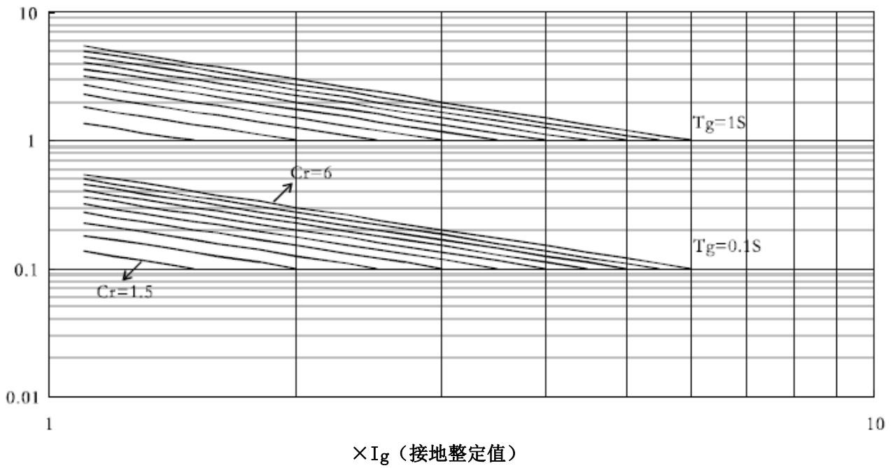
接地保护
