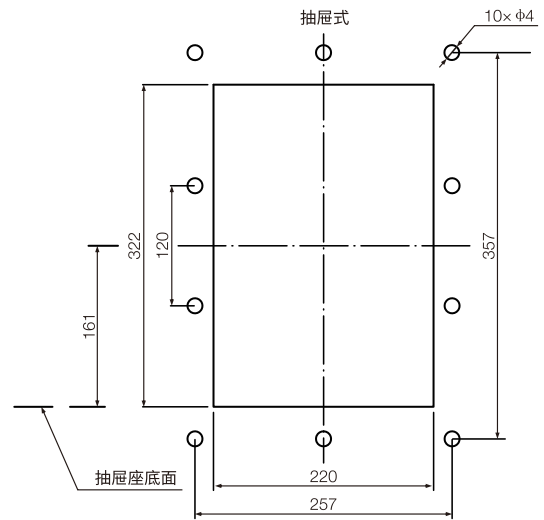
RDW5-1600S抽屉式断路器面板开孔尺寸
