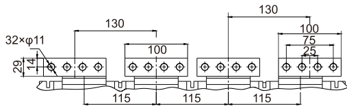
2900-3200 (4P) 水平接线
