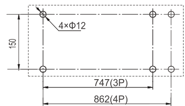
安装尺寸示意图
