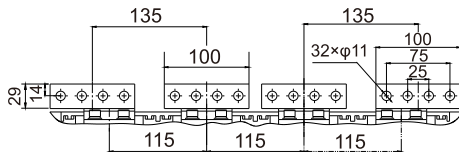
2900-3200 (4P) 水平接线
