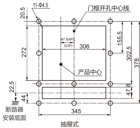
RDW5-2500H抽屉式断路器面板开孔尺寸
