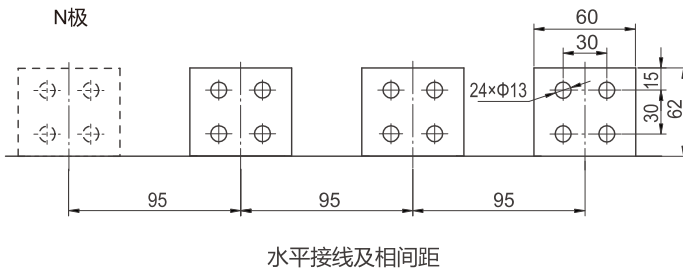
水平接线及相间距
