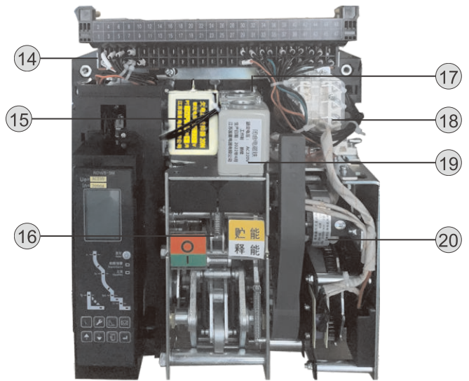
断路器本体
