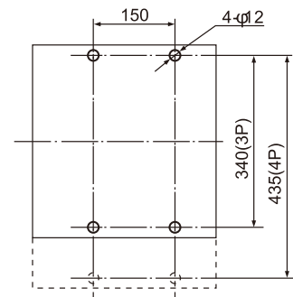
安装尺寸示意图
