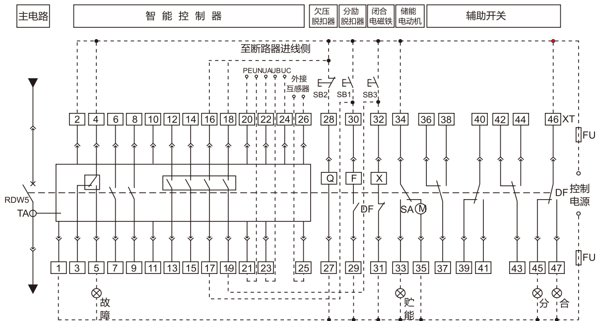
RDW5-1600S,2000-6300S/H带重合闸功能断路器控制回路接线图
