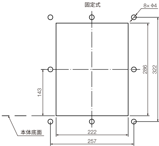
RDW5-1600S固定式断路器面板开孔尺寸
