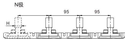
垂直接线及相间距
