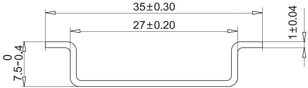
图2 安装轨尺寸
