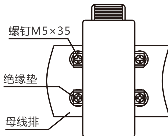
图5 母线固定
