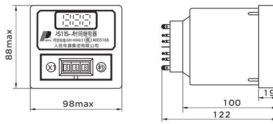
图4 JS11S-J(原JS11J/JS114)外形尺寸
