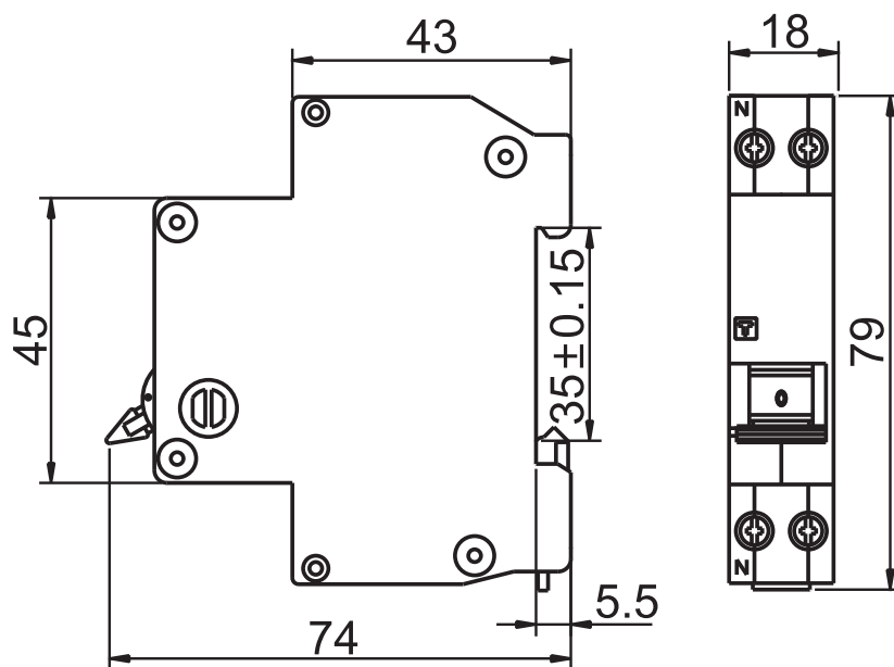
剩余电流动作断路器的外形、安装尺寸图
