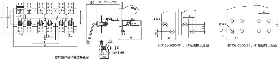
HD13s BX中央旋转操作机构刀开关外形及安装尺寸见图4、表4
