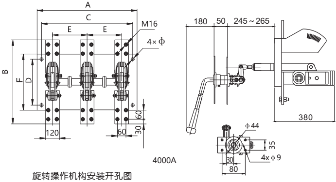
HD13s BX中央旋转操作机构刀开关外形及安装尺寸见图5、表5
