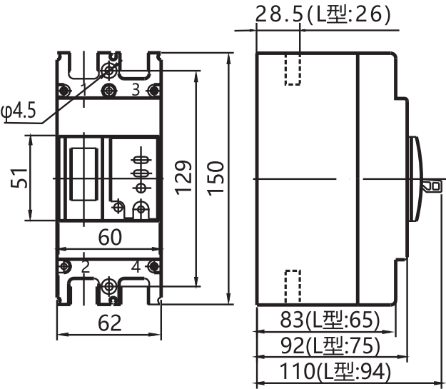
图8a RDM1L-125M/2300
