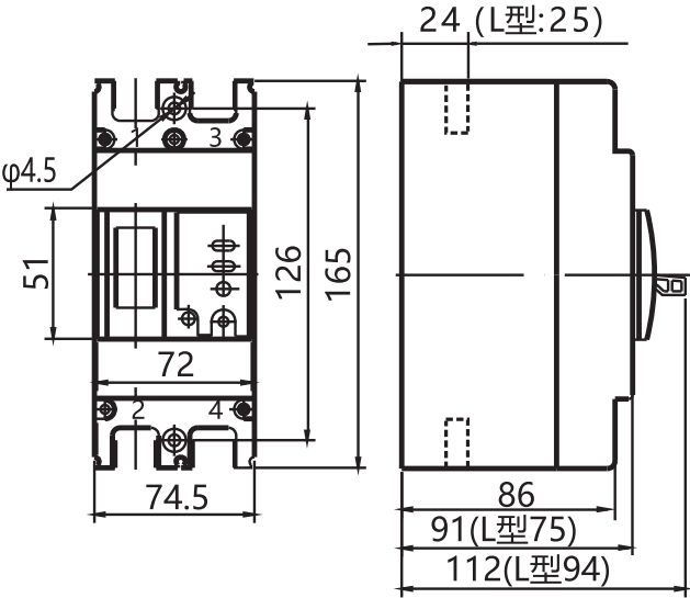
图8b RDM1L-250M/2300
