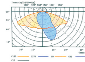
配光曲线
